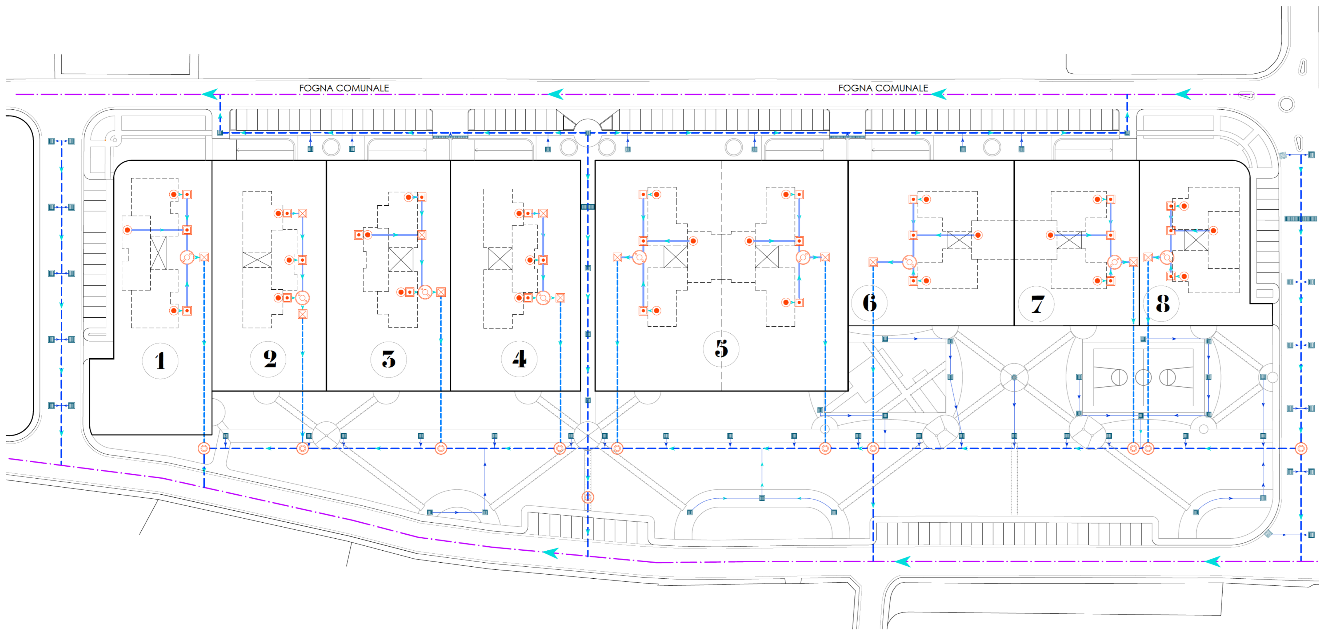
SCHEMA RETE FOGNARIA - scala 1 : 500
