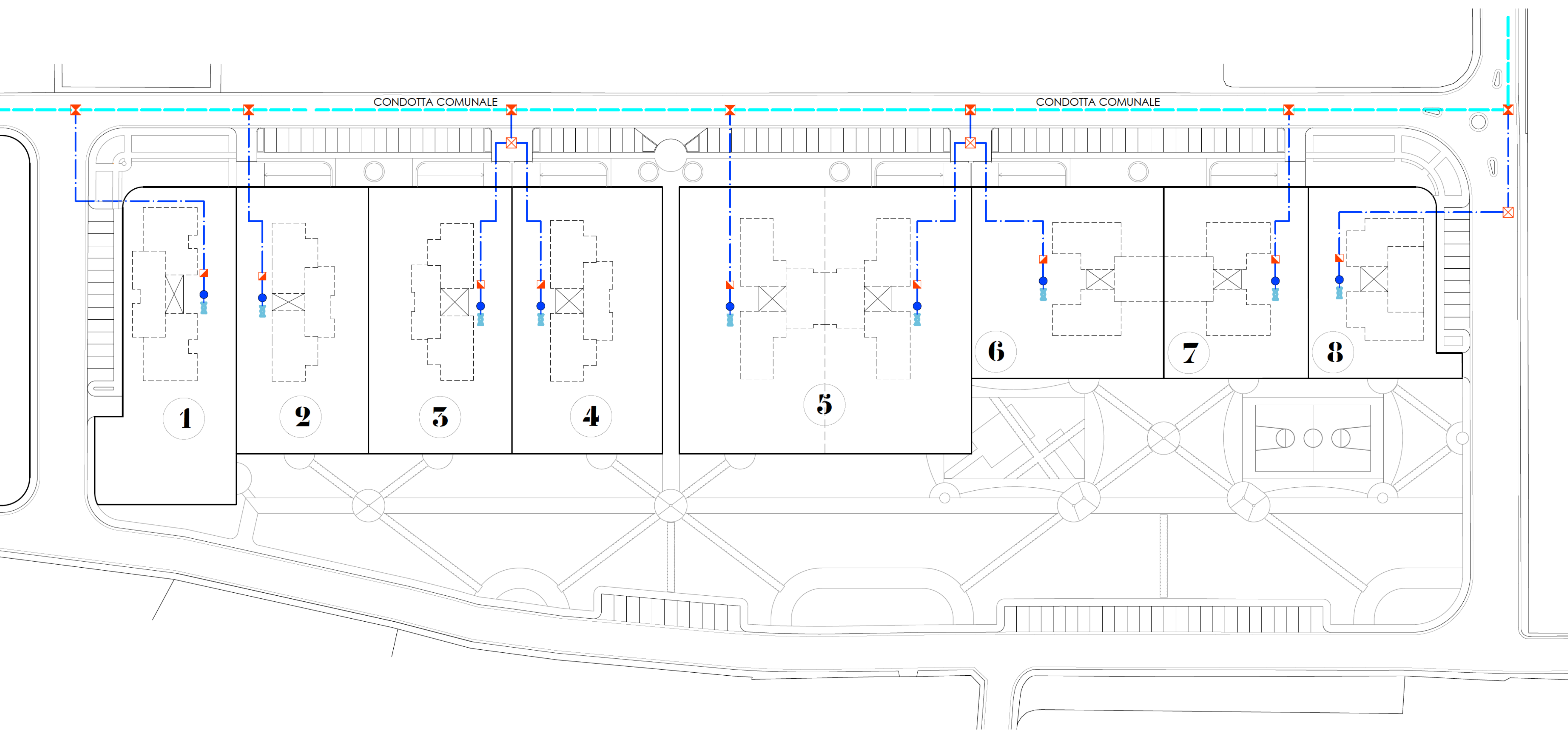
SCHEMA RETE IDRICA - scala 1: 500
