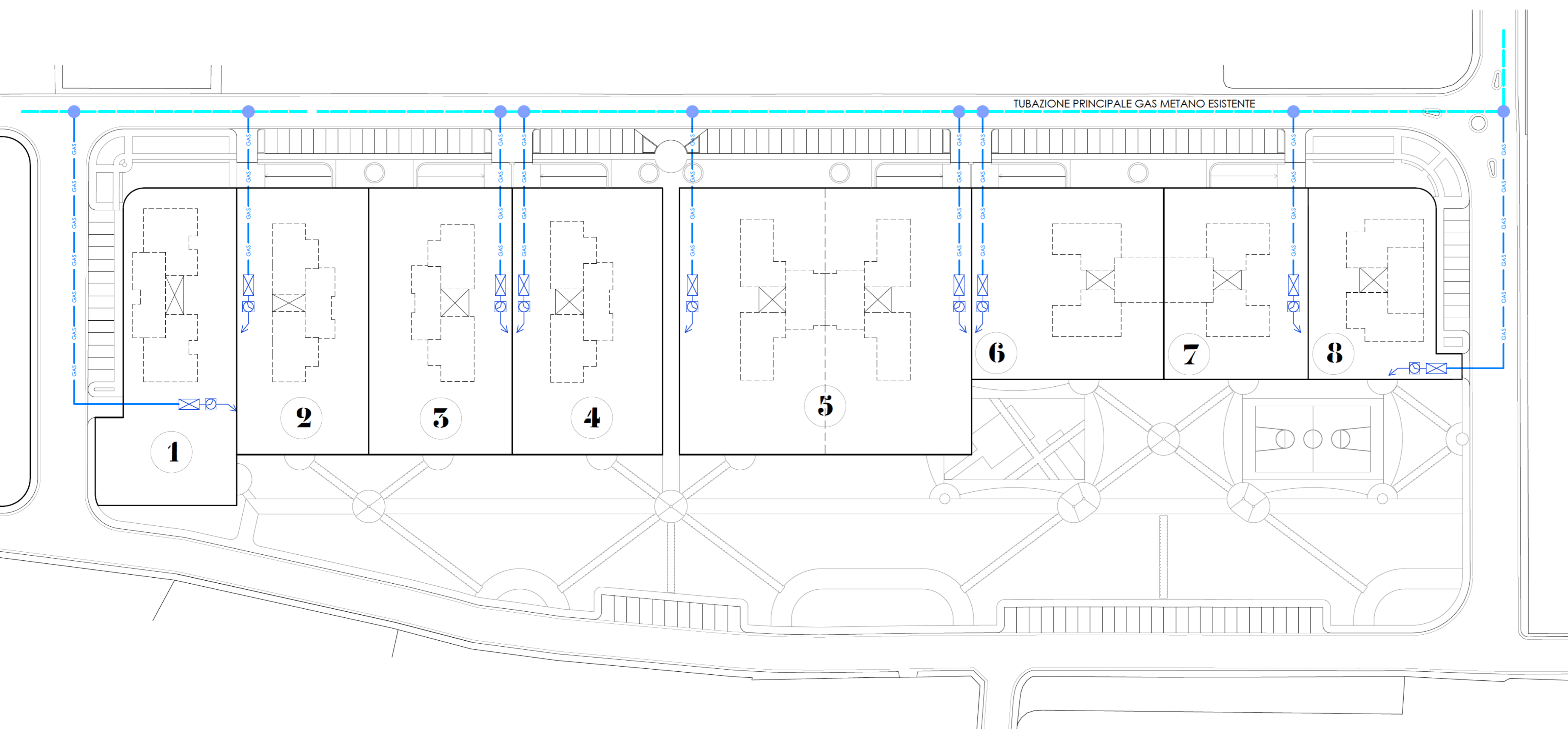
SCHEMA RETE GAS - scala 1: 500
