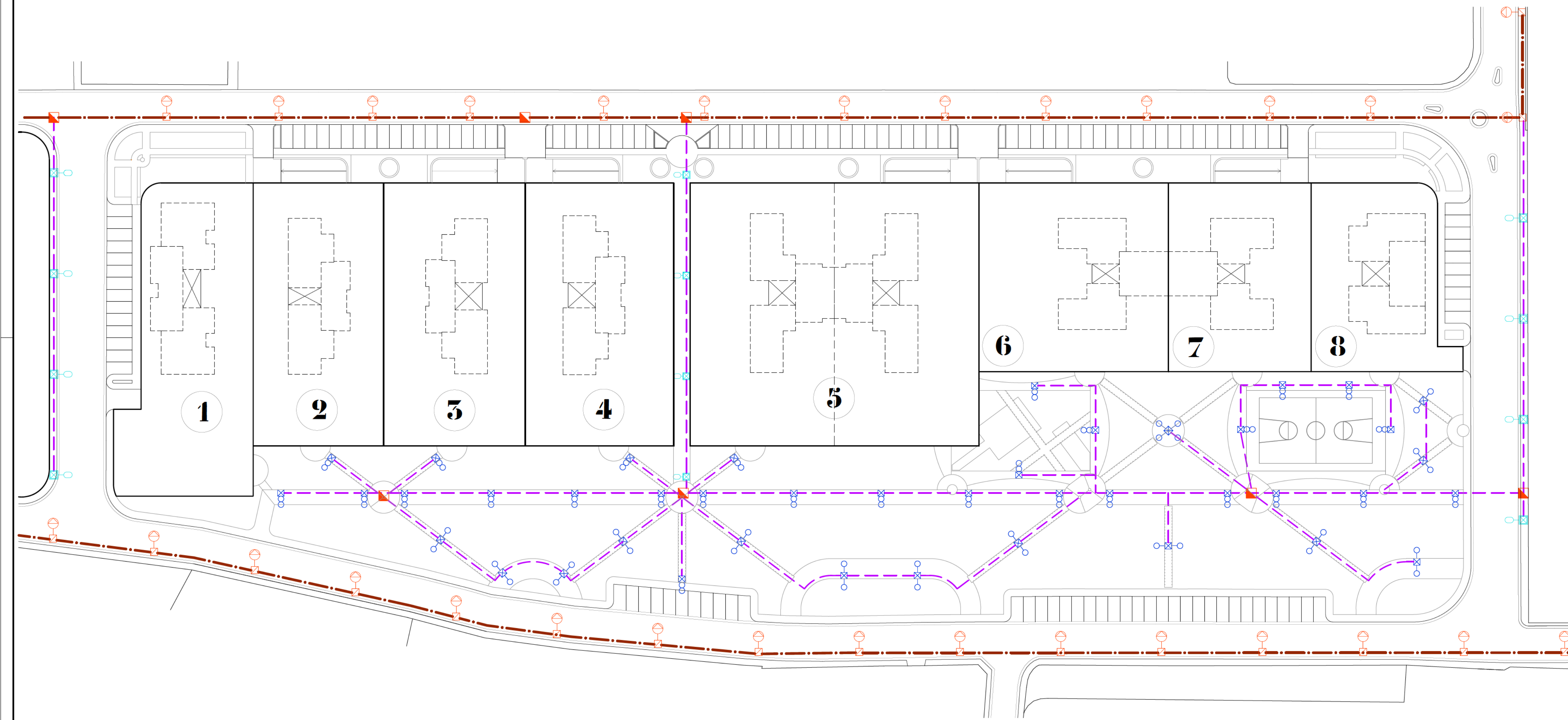
SCHEMA RETE ILLUMINAZIONE - scala 1: 500
